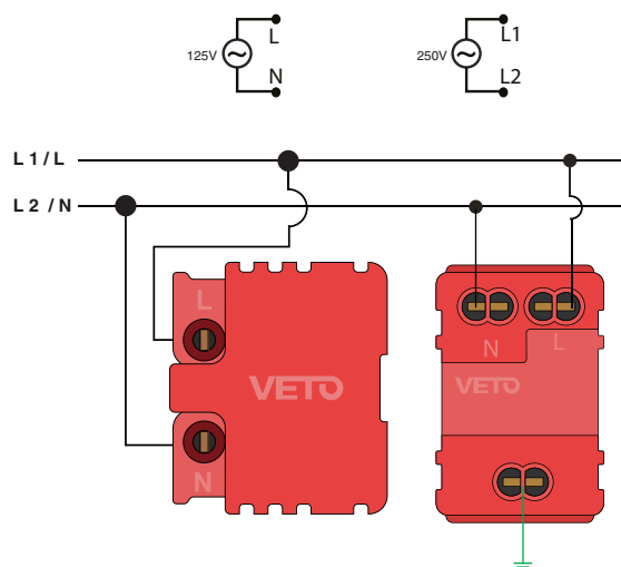
Diagrama de Instalación Base de carga USB
