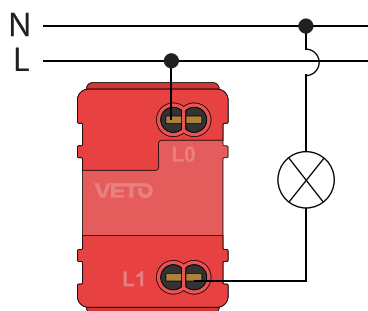
Diagrama de instalación Interruptor
