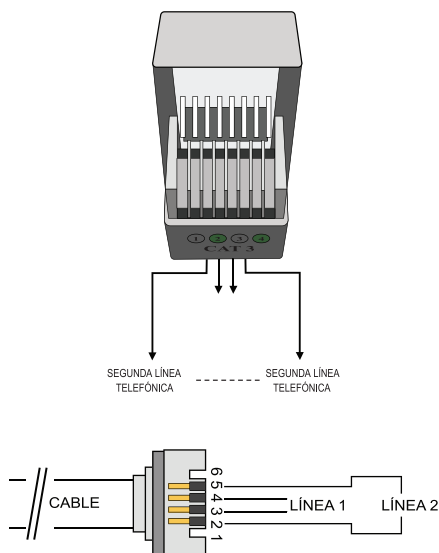
Diagrama de Instalación Jack telefónico
